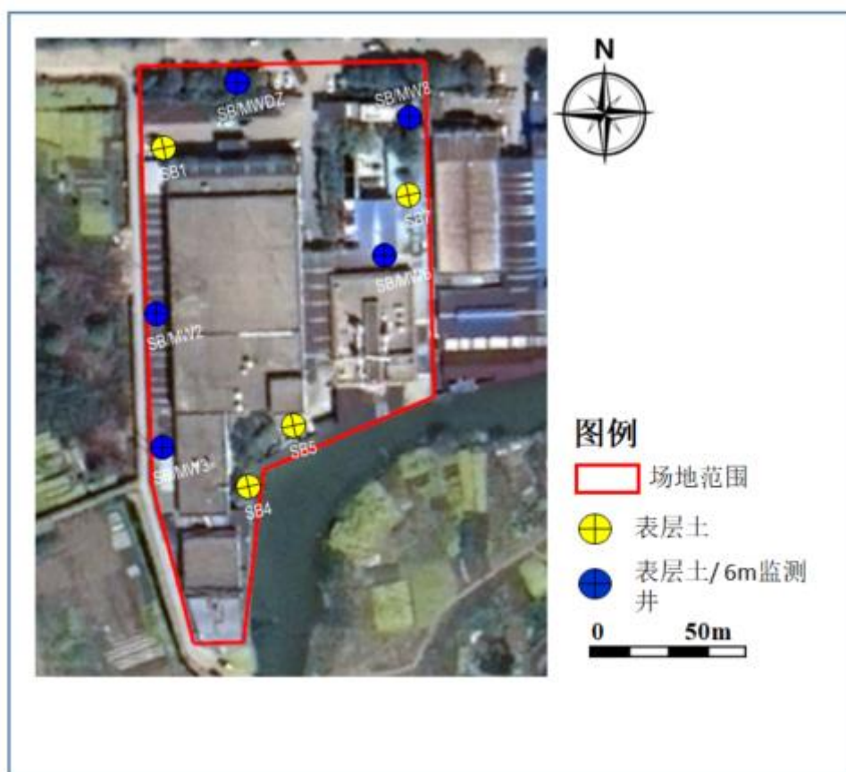
图 7.2 地块内监测点位汇总示意图
