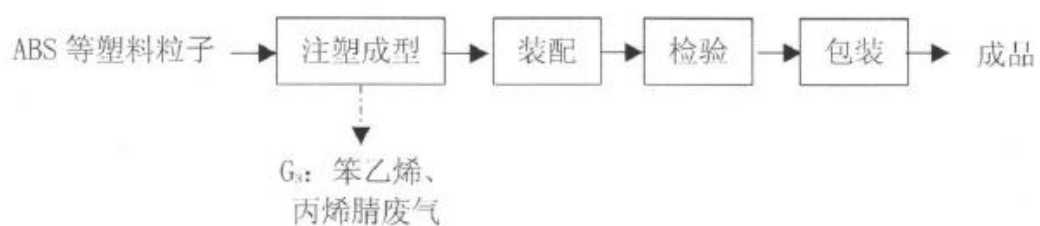
图 4.2 工艺流程图
