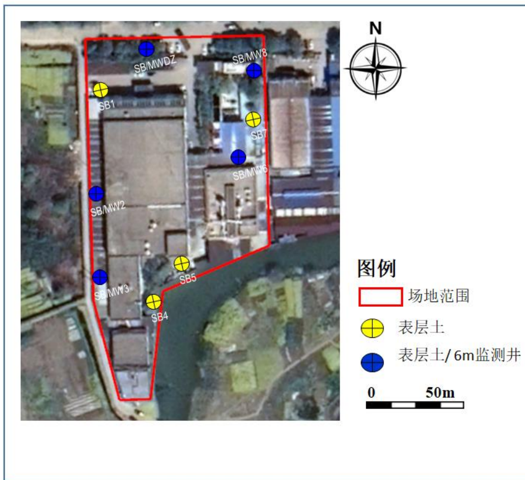
图 4.3 厂区平面布置图
