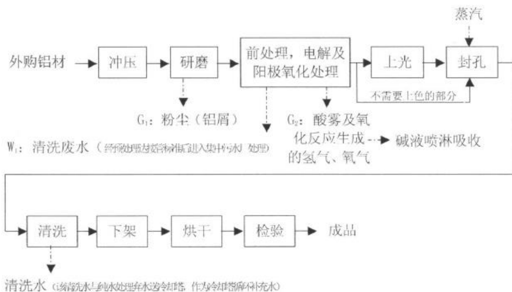
图 4.1 工艺流程图
